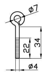
Bolt/Eyelet Stud Bolt-04
