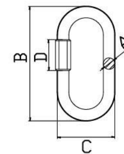
Quick Link LQ01
